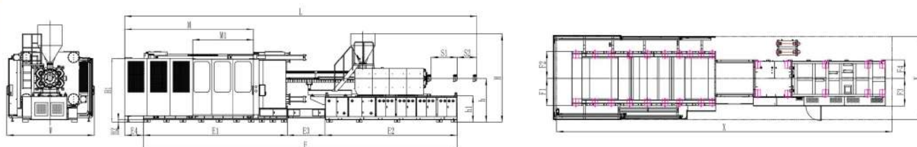
机型尺寸 Principal Dimensions
